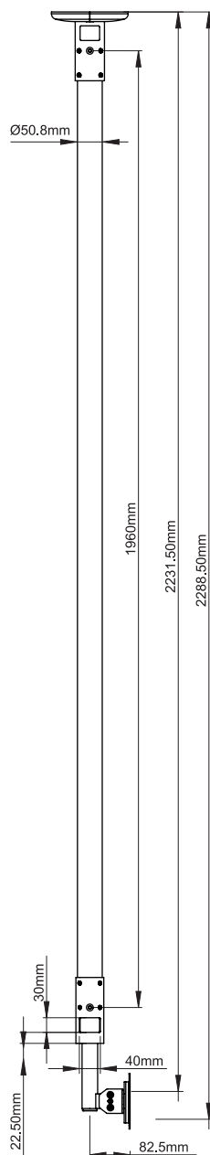
BT7553-200
