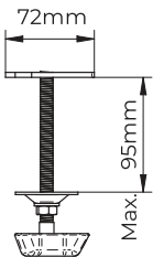
Grommet Clamp
