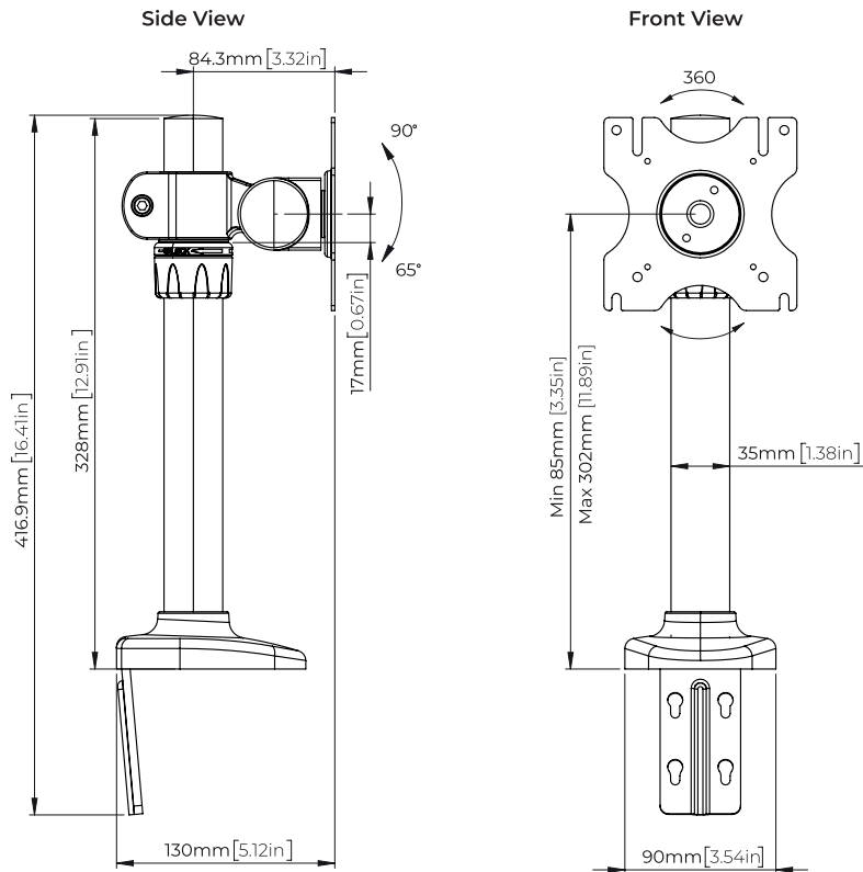
Grommet Clamp
